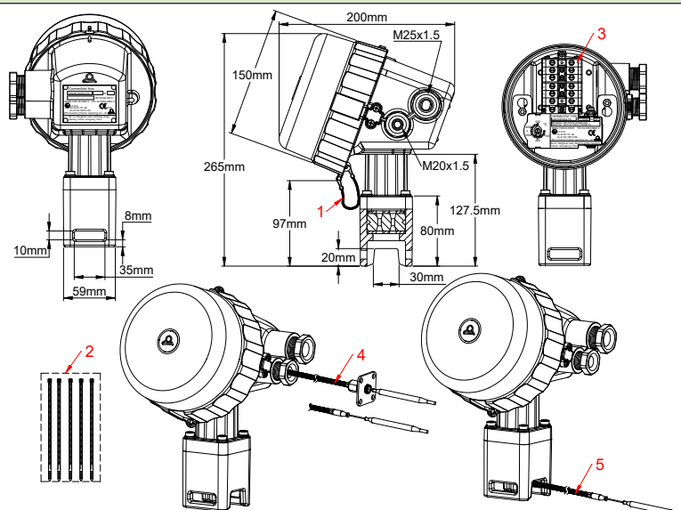
1 : Chainette de couvercle, 2 : Scellés rouges, 3 : Jeu de borniers, 4 : Sortie du capillaire par presse-étoupe M20, 5 : Sortie du capillaire par le pied de montage sur tube.
