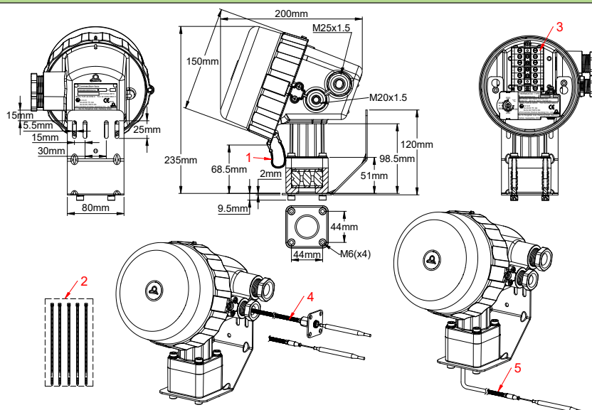
1 : Chainette de couvercle, 2 : Scellés rouges, 3 : Jeu de borniers, 4 : Sortie du capillaire par presse-étoupe M20, 5 : Sortie du capillaire par le pied de montage sur tube.
